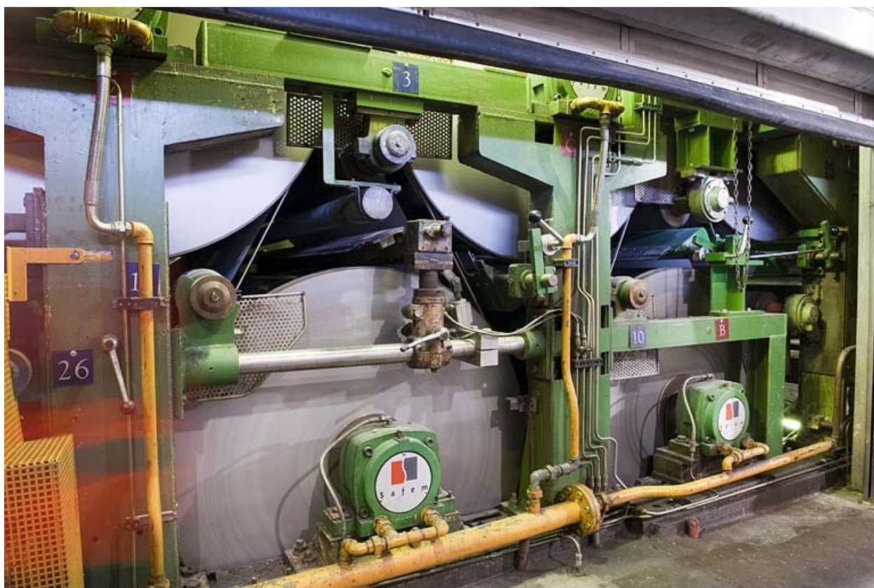
Machine à papier. Vue rapprochée de la partie séchage.
