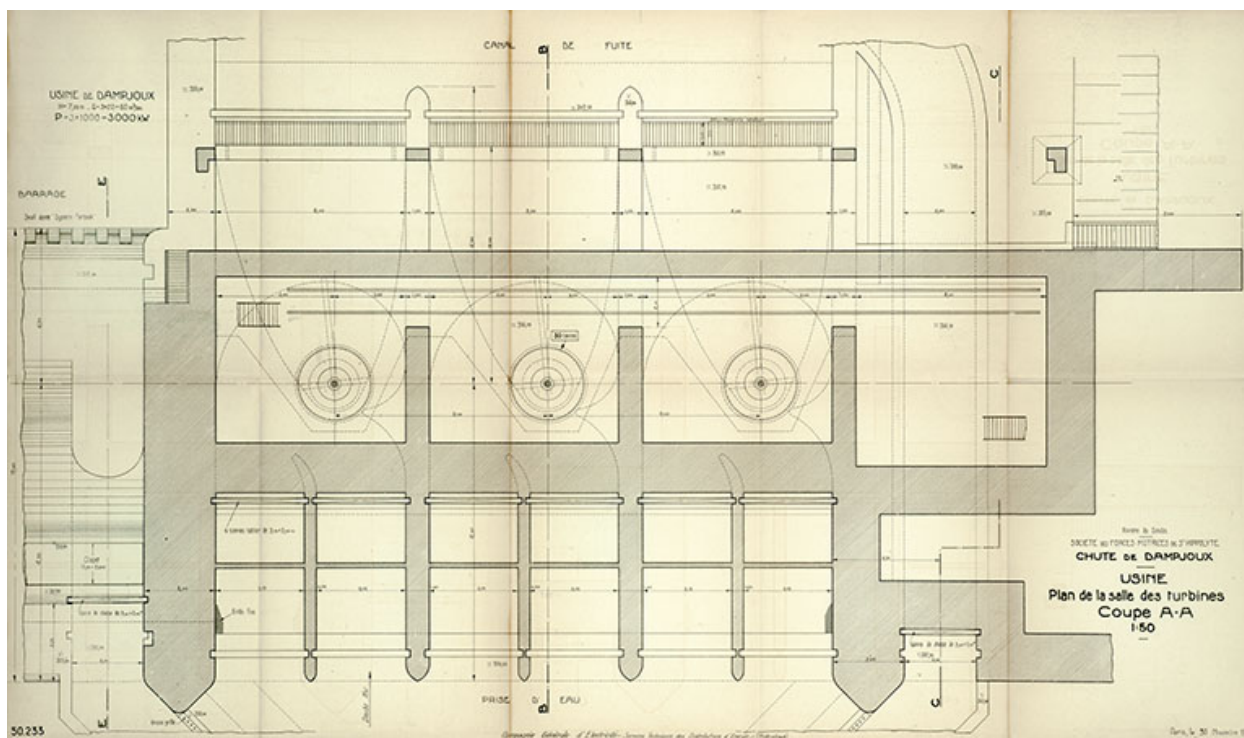
Chute de Dampjoux. Usine. Plan de la salle des turbines. Coupe AA, 1930.
