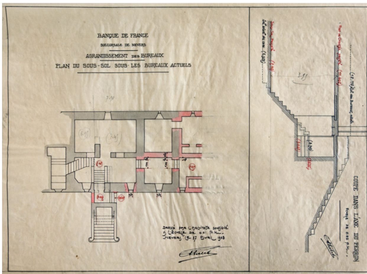
Plan et coupe du sous-sol (7 avril 1908).
