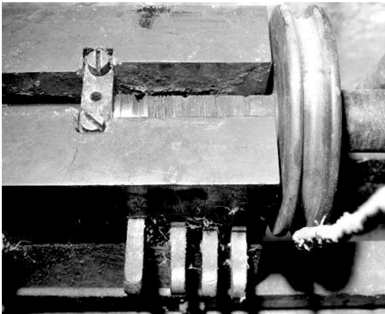
Détail du filetage de l'arbre du tour et des clés de sélection.
