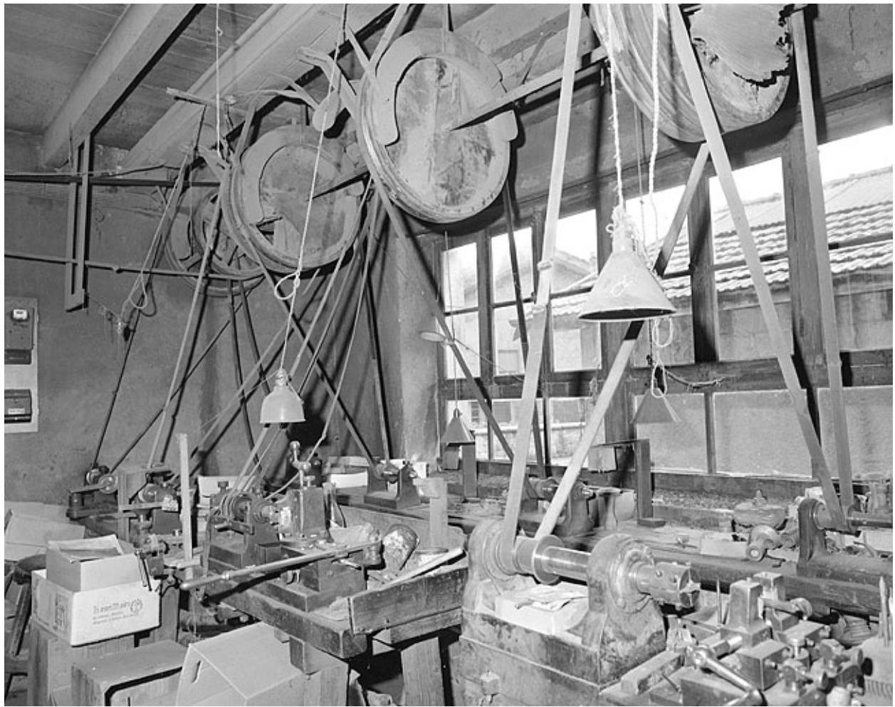
Partie de l'atelier utilisée pour la finition des pipes.
