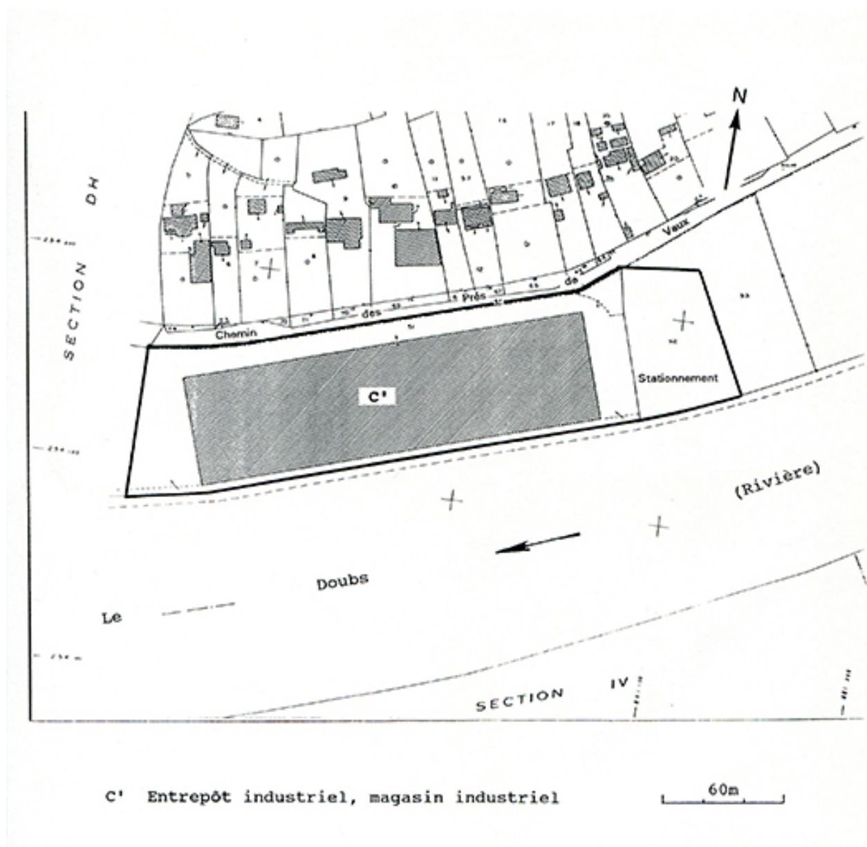
Plan-masse de la partie orientale du site industriel (usine C). Extrait du plan cadastral, 1982, section DH, 1/1 000 réduit à 1/2 000.
