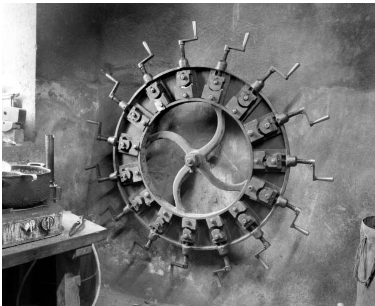
Usine de tabletterie (usine de pipes) Ropp puis Waille, Saint-Claude (5 rue Saint-Oyend, 51 bis rue de la Poyat) : machine à cintrer les tuyaux en corne.
