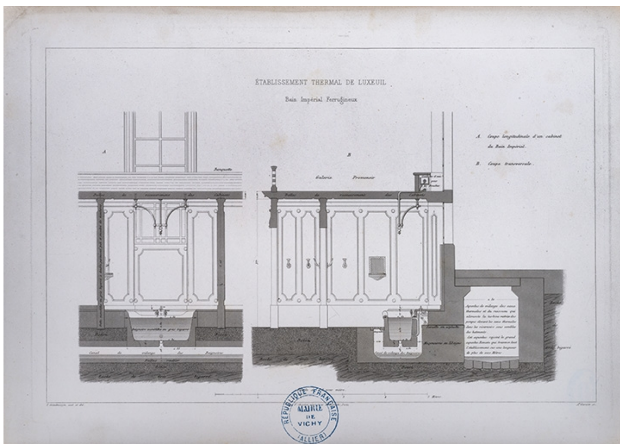
Coupes sur une cabine du Bain impérial ferrugineux.
