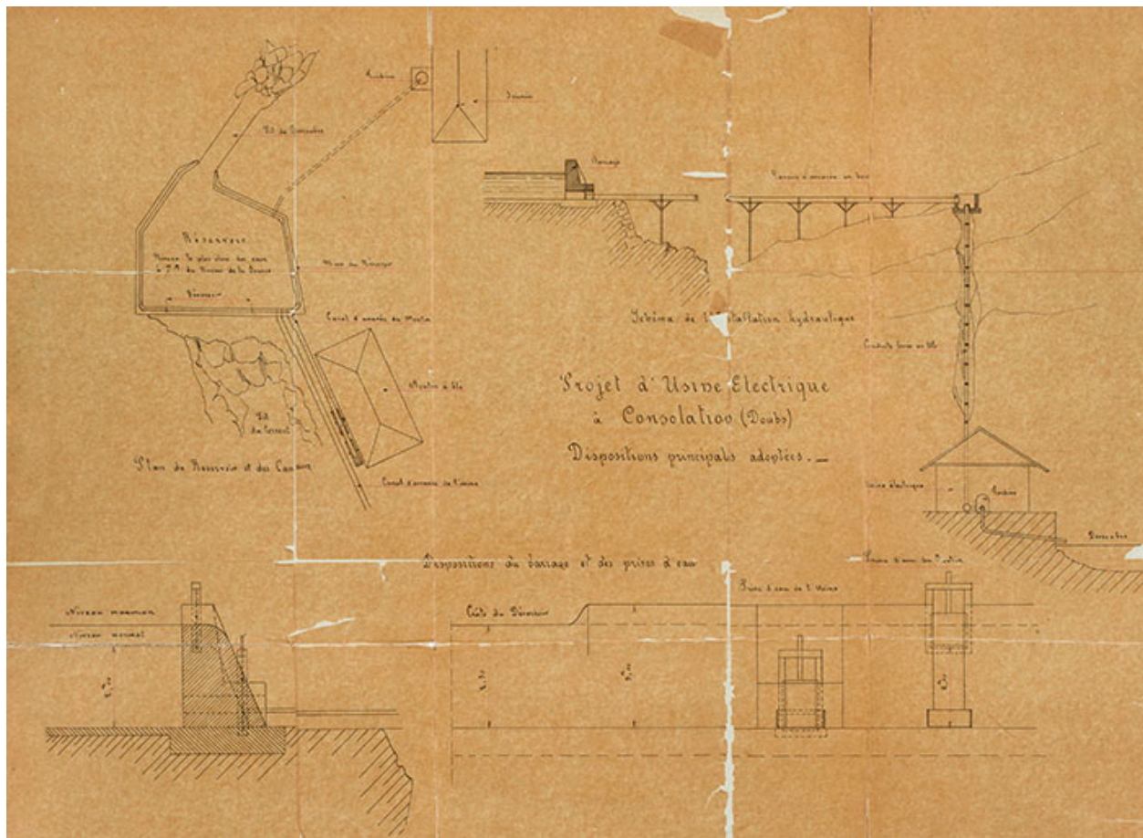
Projet d'usine électrique à Consolation (Doubs), s.d. [1895].
