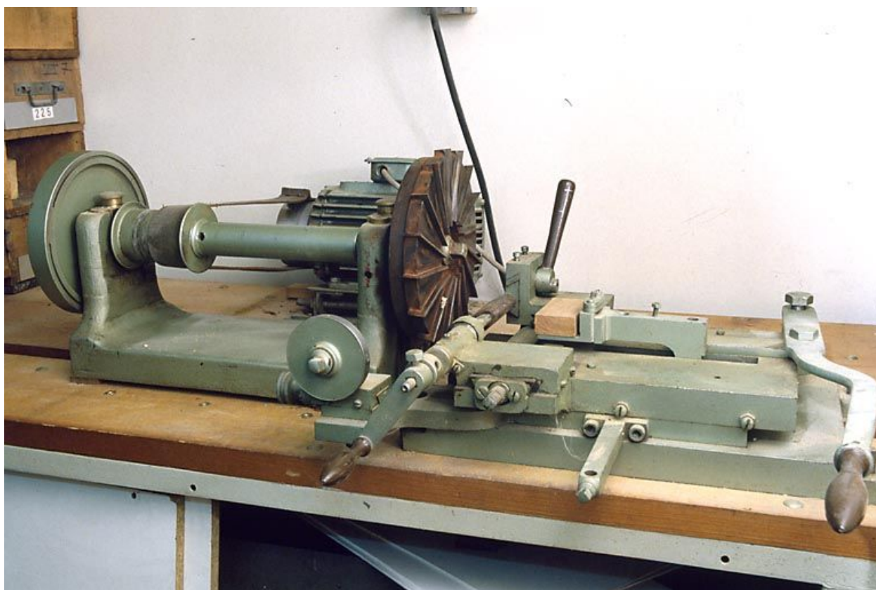
Machine à fraiser dite machine à ovaliser ou varlope.
