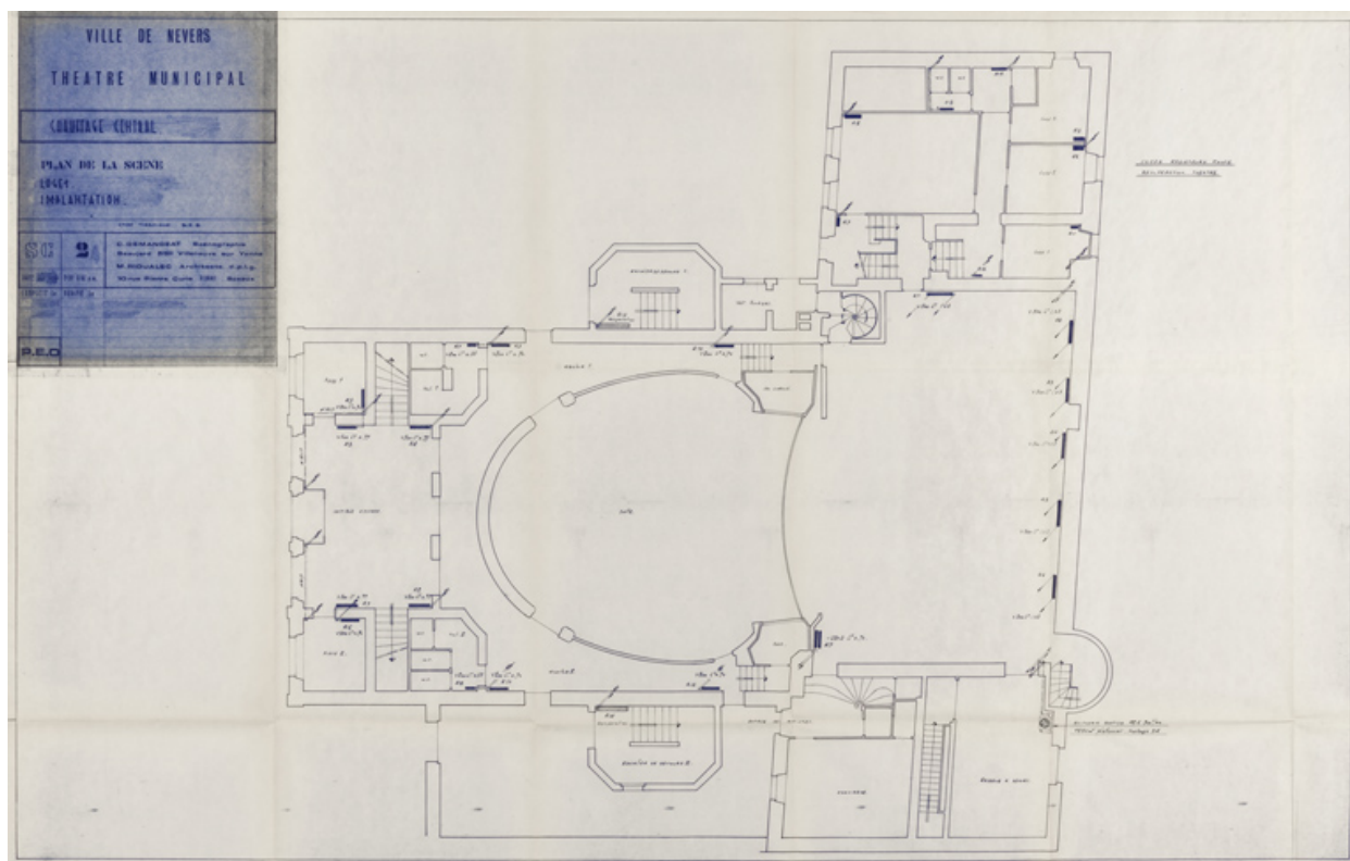
Ville de Nevers. Théâtre municipal. Chauffage central. SC 2. Implantation. Plan de la scène. Loges. Octobre 1978.
