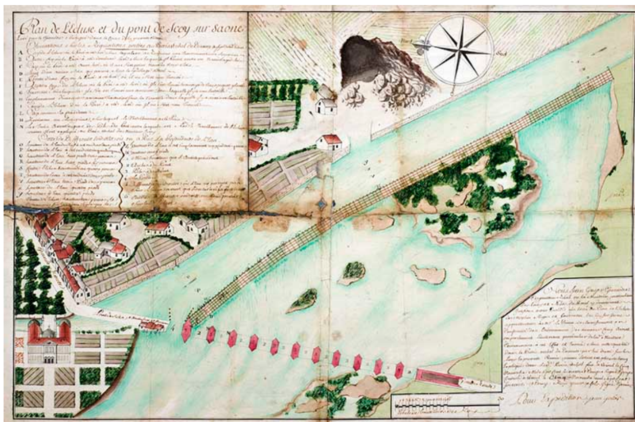
Plan du pont de Scey-sur-Saône, avec le château et une partie de son jardin (1772).
