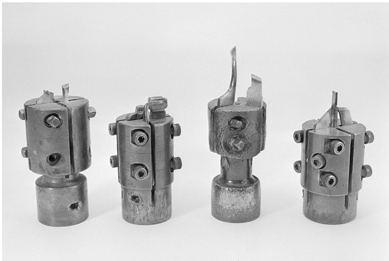
Détail de quatre outils de coupe.
