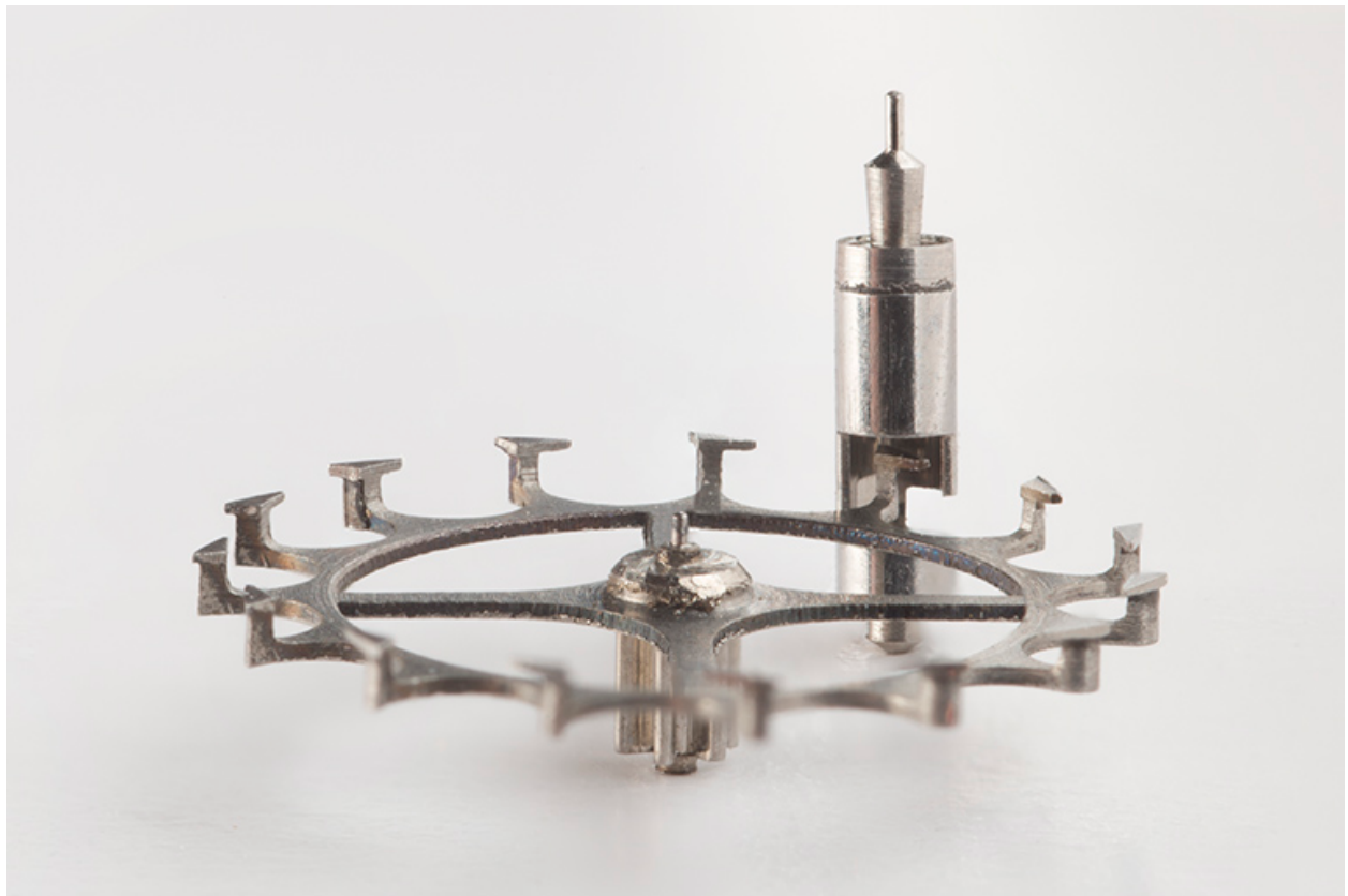
Echappement à cylindre.
