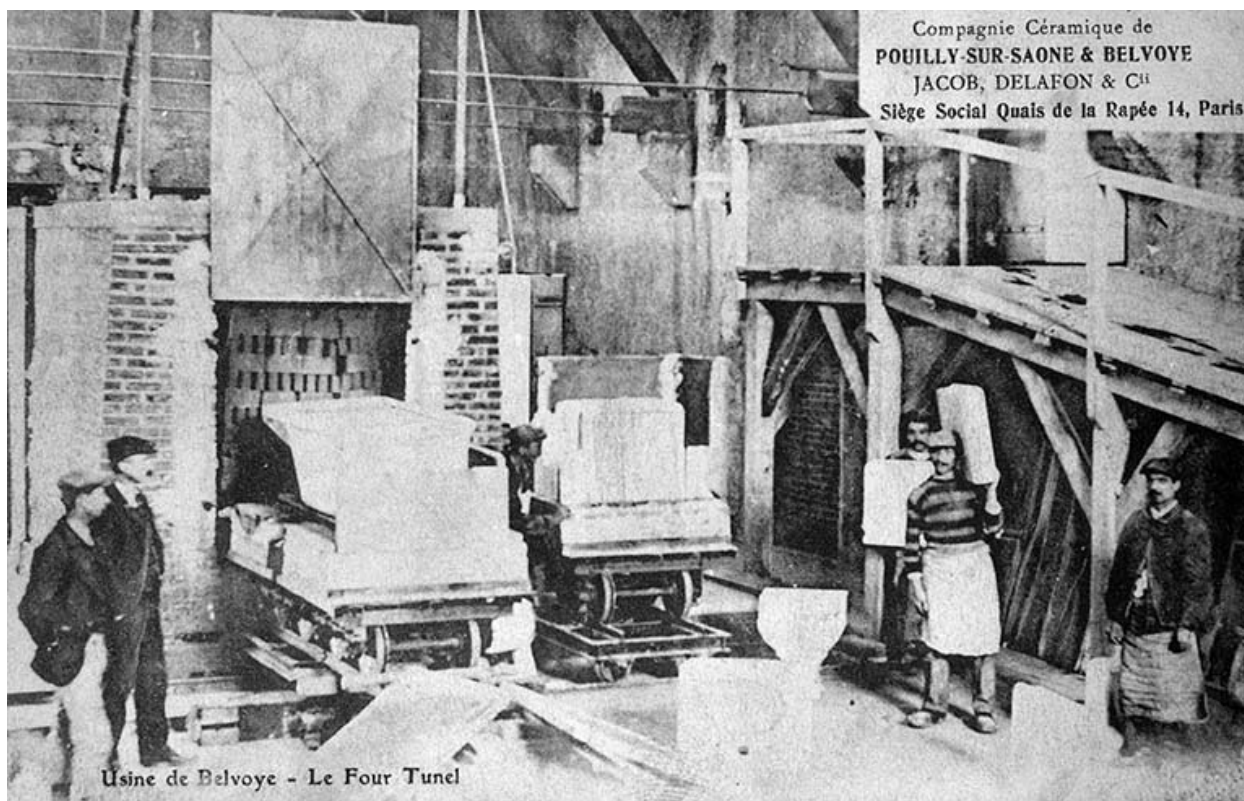
Usine de Belvoye - Le Four Tunel (four Dinz), [limite 19e siècle 20e siècle, entre 1899 et 1906].
