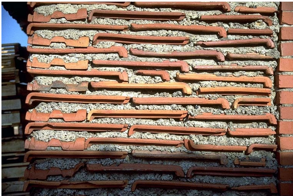
Atelier de fabrication : tuiles en gros oeuvre.
