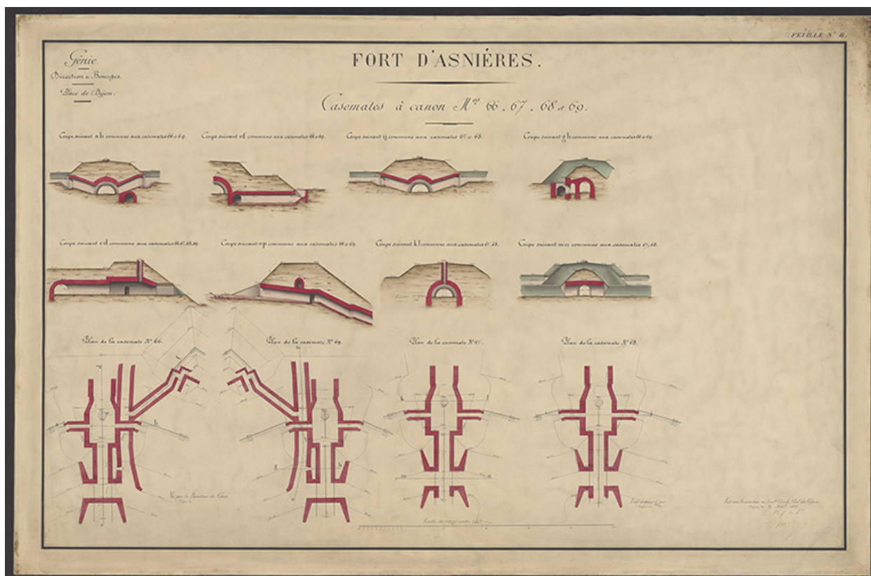
Fort d'Asnières. Casemates à canons n° 66, 67, 68 et 69. 1885.
