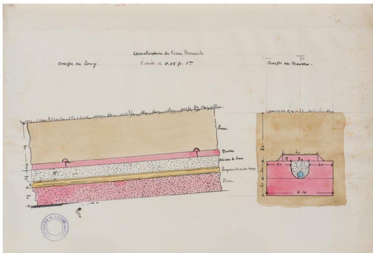
Coupes sur une canalisation (1895).
