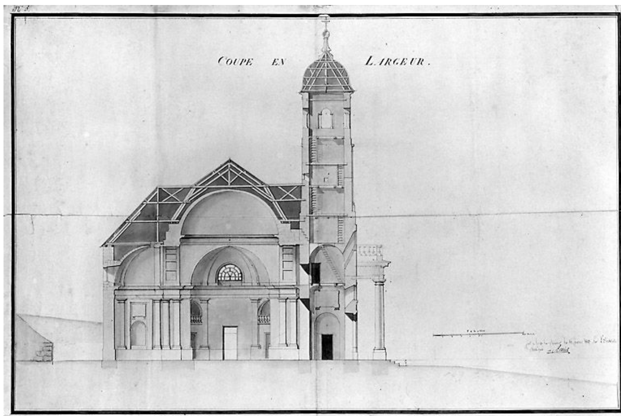
Coupe en largeur, 1813. Dessin (plume, lavis), 14 février 1813, échelle approximative 1:90.
