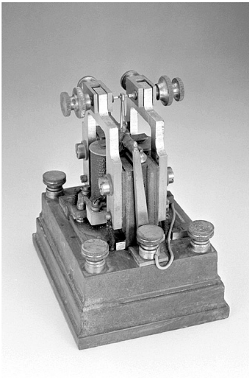
Vue latérale de l'un des relais sans couvercle.
