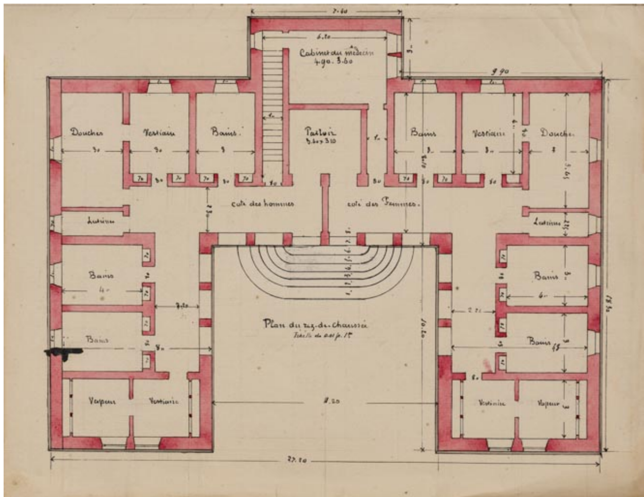
Plan du rez-de-chaussée (1895).
