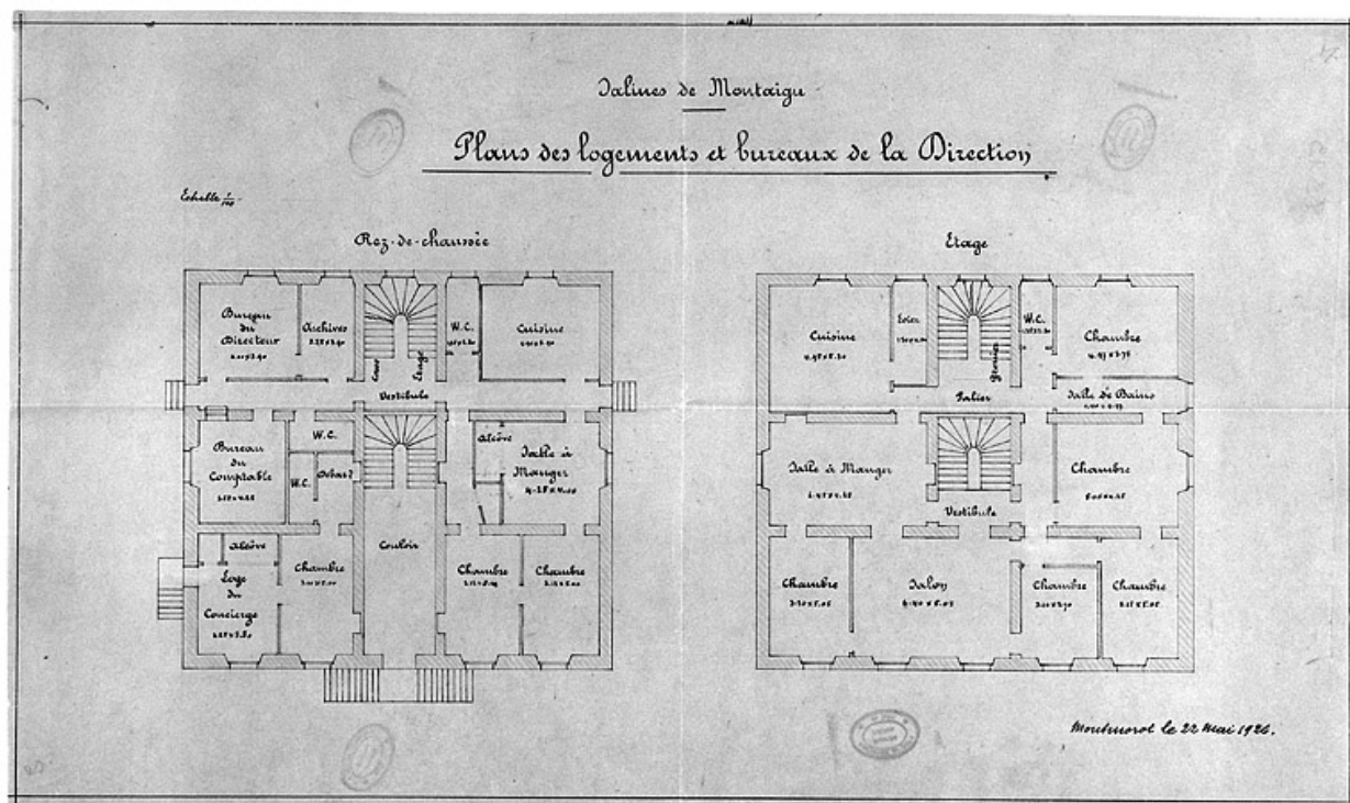
Salines de Montaigu. Plans des logements et bureaux de la Direction.
