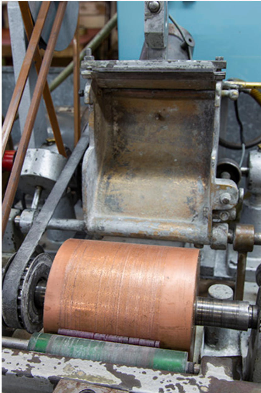
Atelier de taille du rubis : l'une des machines à usiner par abrasion.
