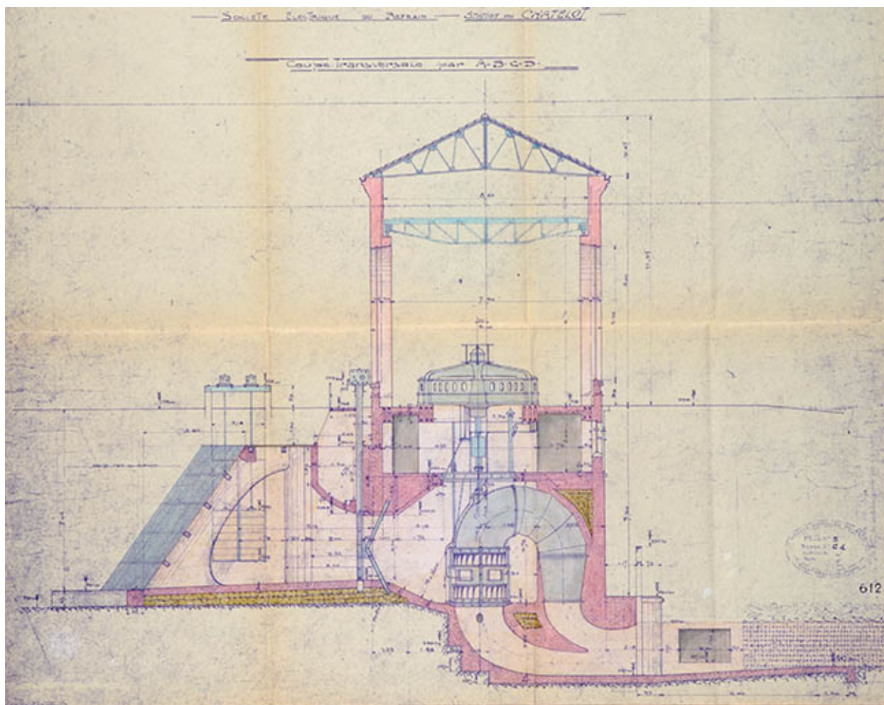
Société Electrique de Belchamp. Station du Chatelot. Coupe transversale de l'usine, pièce n° 10, 1934.
