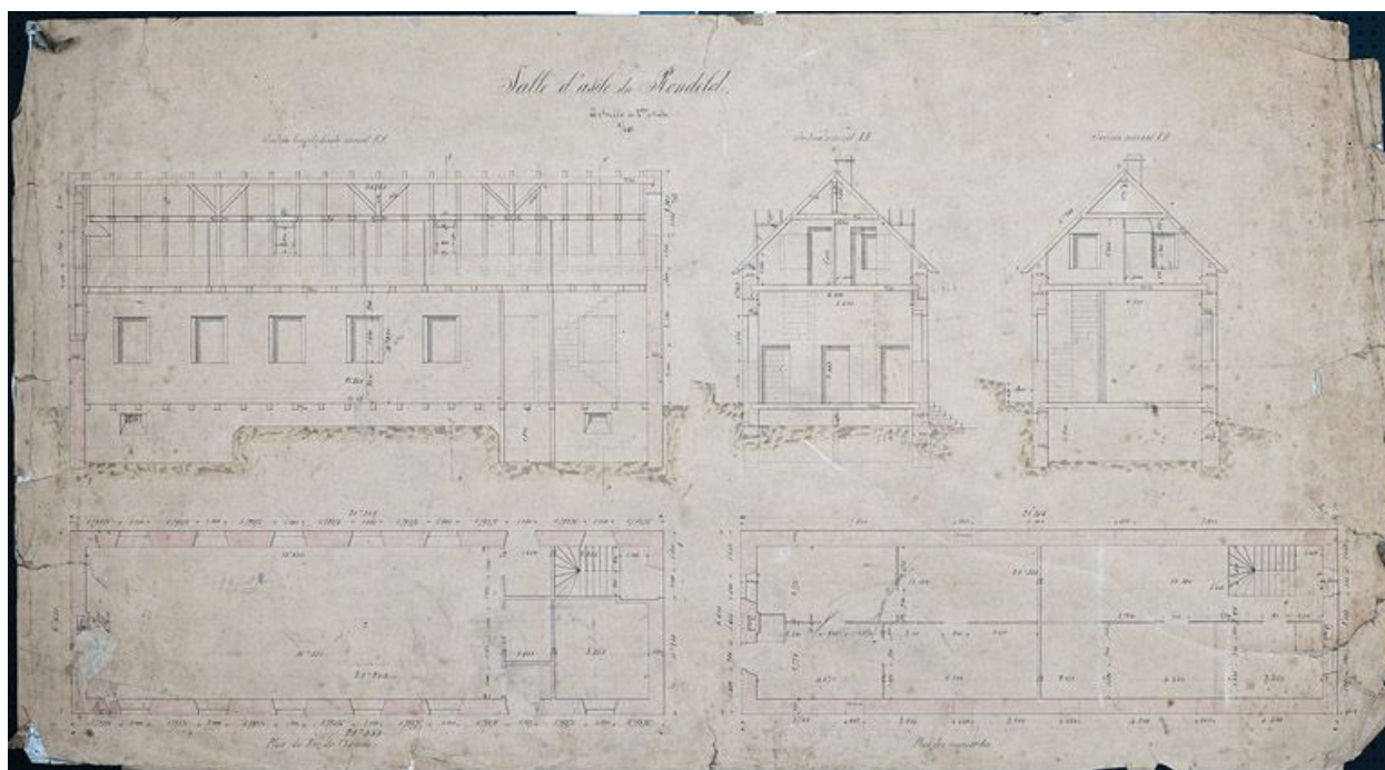
Salle d'asile du Rondelot. Plan, plume, encre, lavis, échelle 1/50, s.d. [fin 19e ou début 20e].
