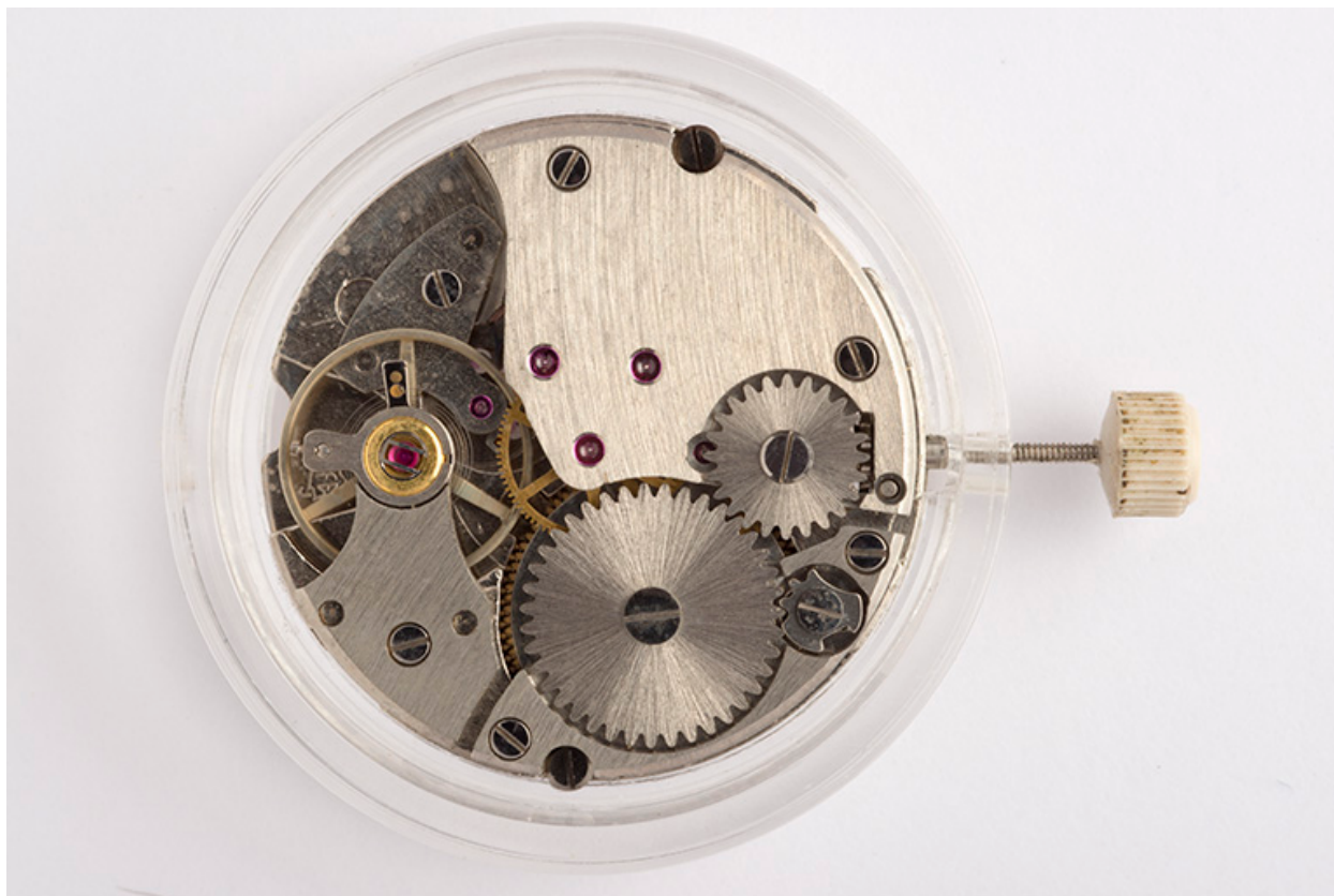
Mouvement de montre France Ebauches FE 140, à Maîche, années 1980.
