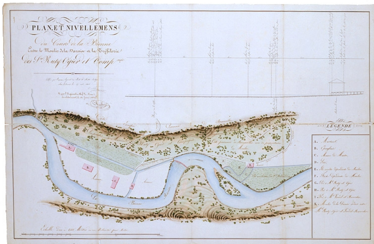
Plan et nivellemens du Cours de la Bienne entre le Moulin de la Daraise et la Tréfilerie des Srs Rutly Ogier et Comp.
