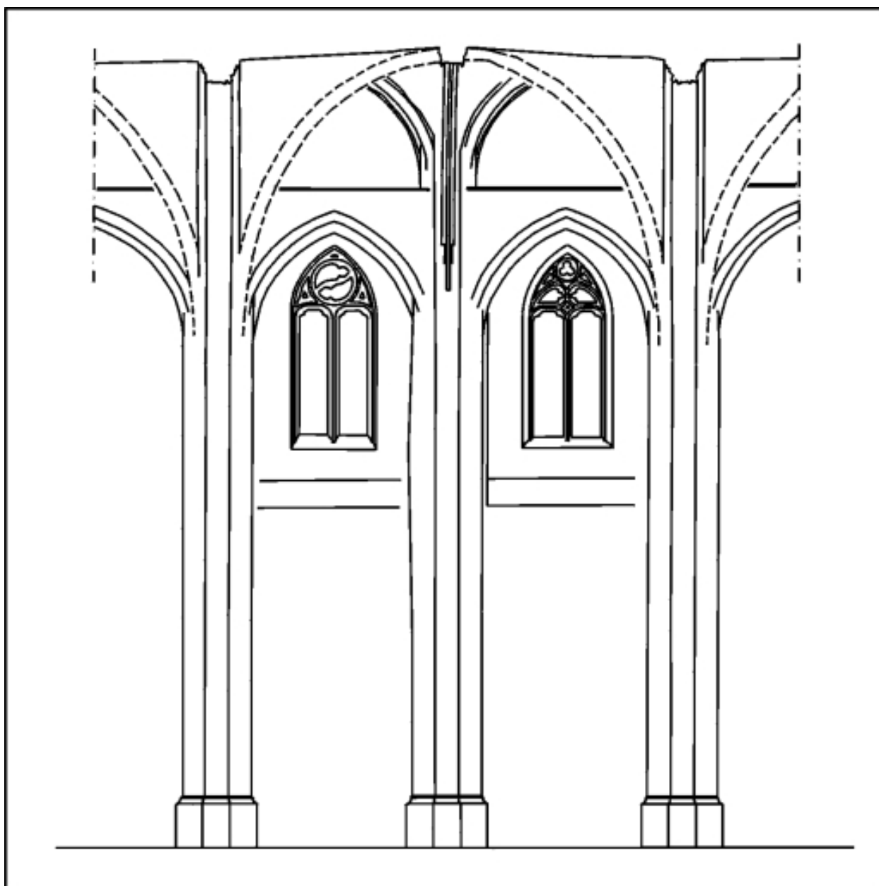
Restitution photogrammétrique d'une partie de la coupe longitudinale.
