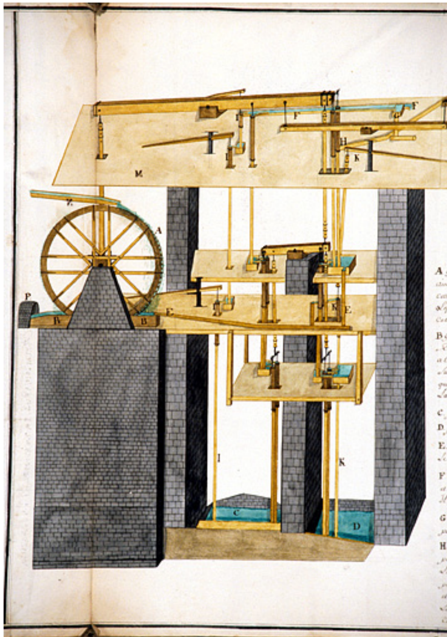
Machines Hydrauliques Qui Elèvent Les Eaux salées et douces du puit à Muire [détail du système d'élévation], 1756.
