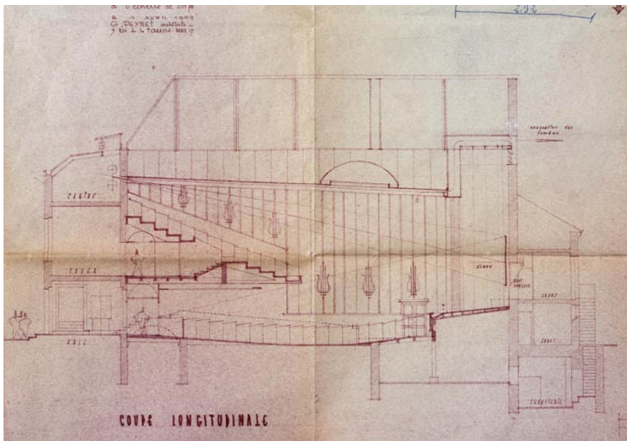
Cinéma Rex à Beaune. 800 places. Avant projet. [Détail :] Coupe longitudinale. 1er avril 1951.
