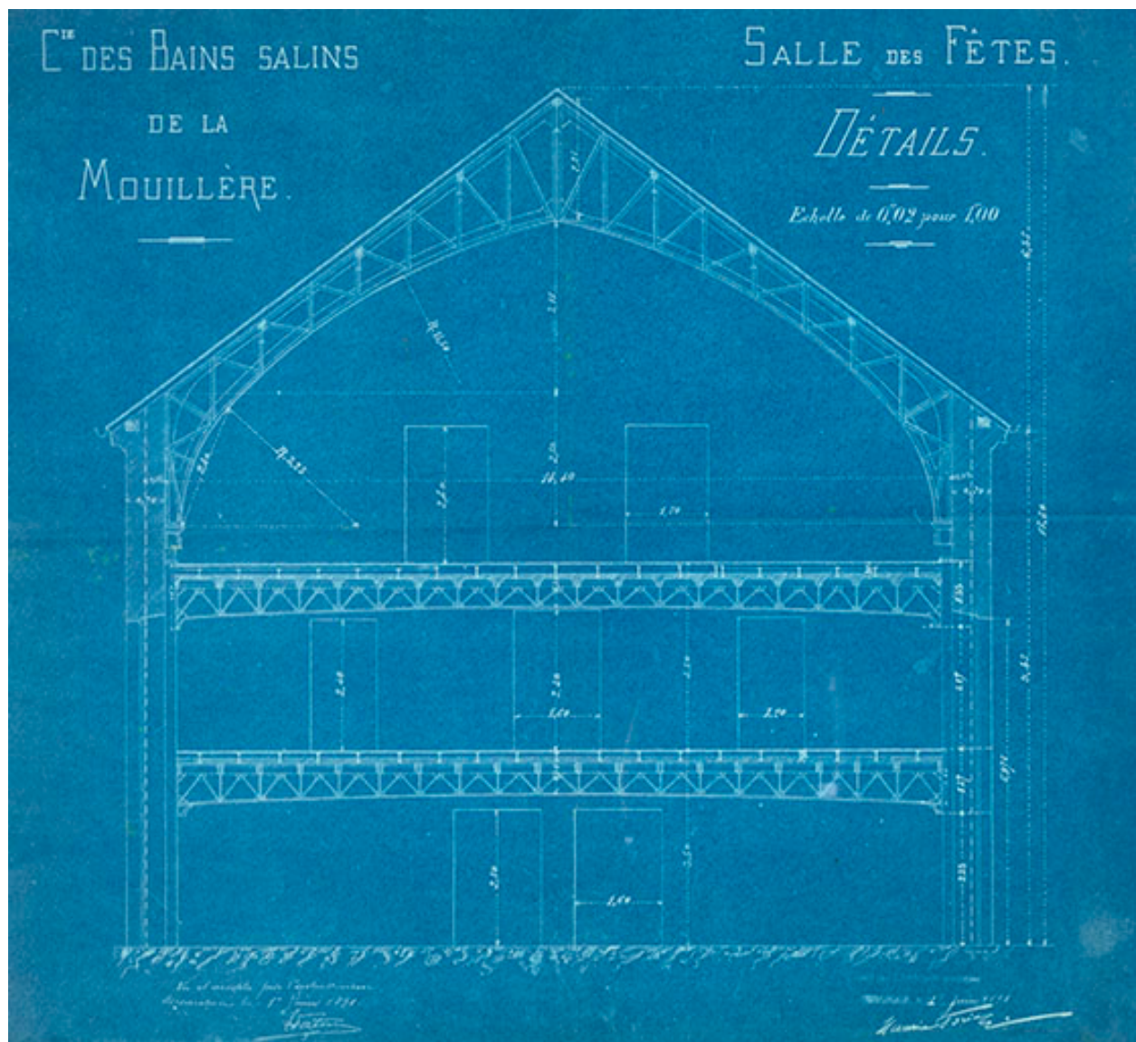
Coupe transversale (1891).
