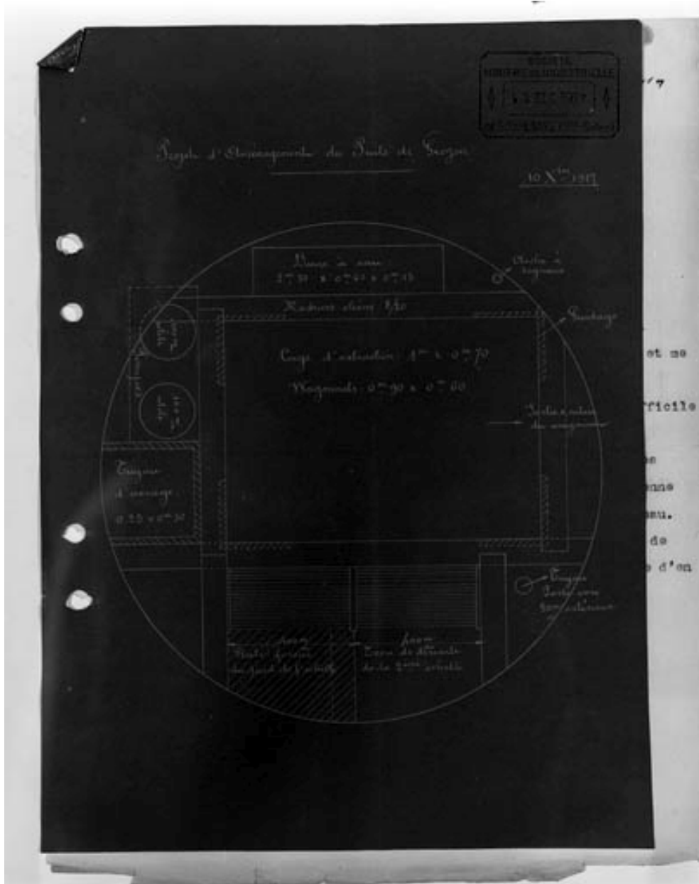
Projet d'aménagement du puits de Grozon.
