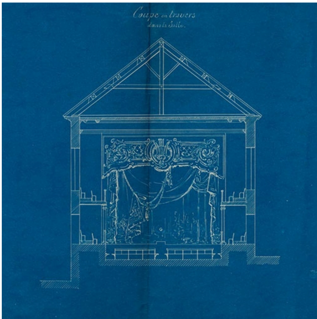
1721. Ville de Semur. Théâtre. Projet d'aménagement. [Détail :] Coupe en travers dans la salle. S.d. [1903 ?].
