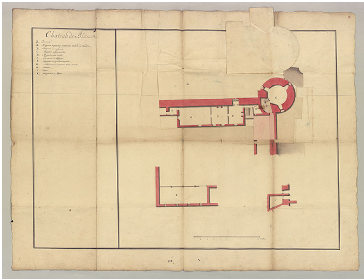
Fol. 18 Château de Blamont : plans (magasin pour 10,000 milliers de poudre) [vue 2].
