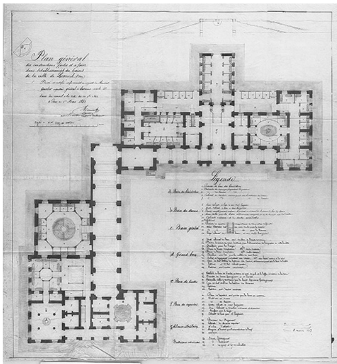
Projet de Bain spécial ferrugineux, plan du rez-de-chaussée (1er mars 1843).
