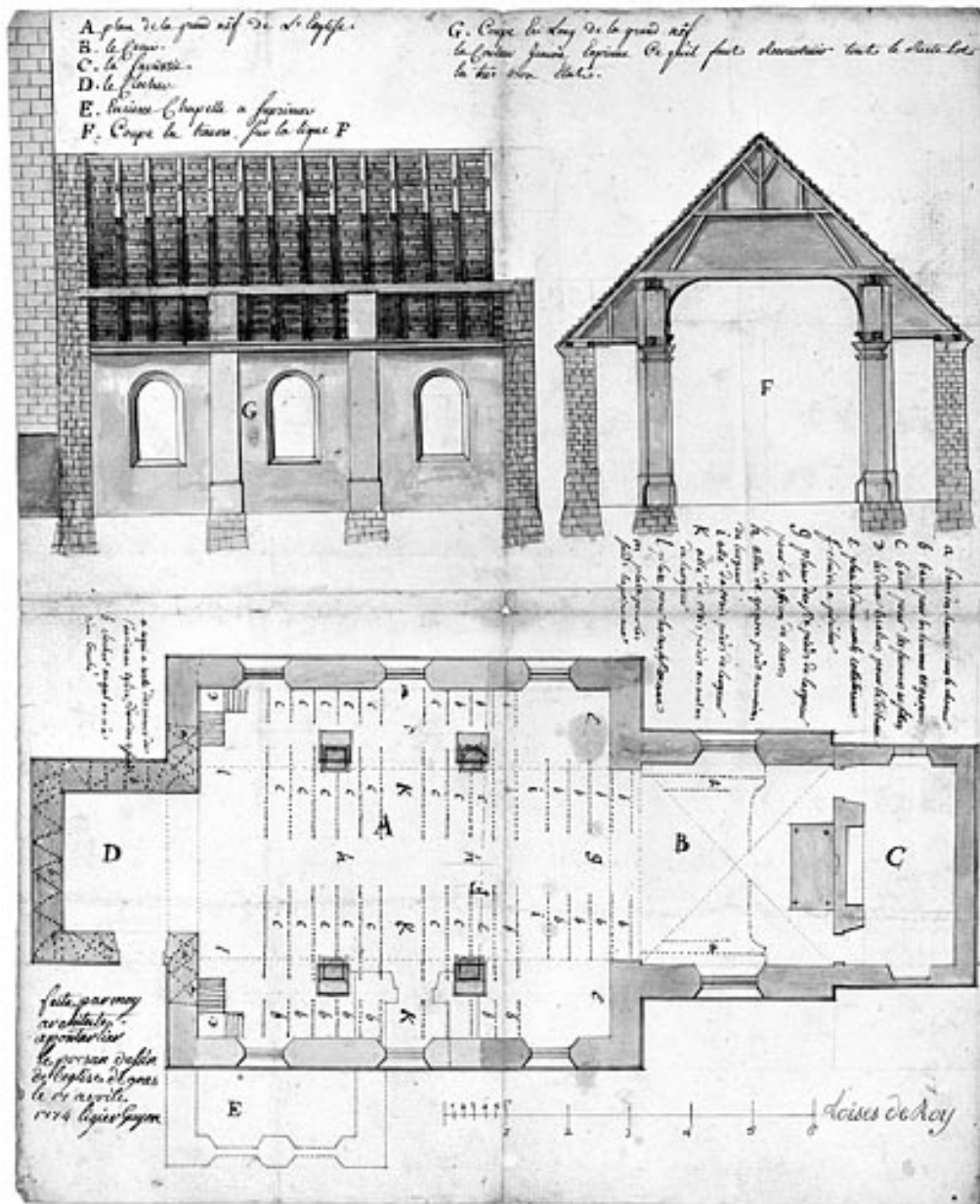
Plan et coupes de l'église.
