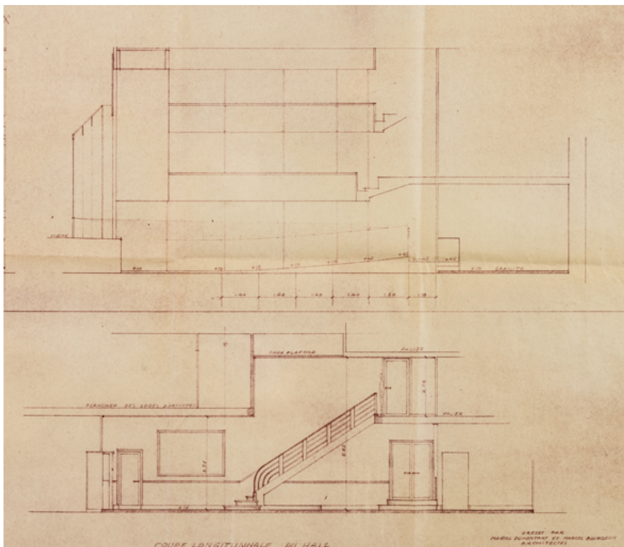
Théâtre municipal. Transformations. Coupes [détail]. 18 mai 1931.
