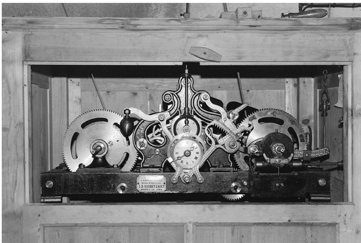
Mécanisme de l'horloge.
