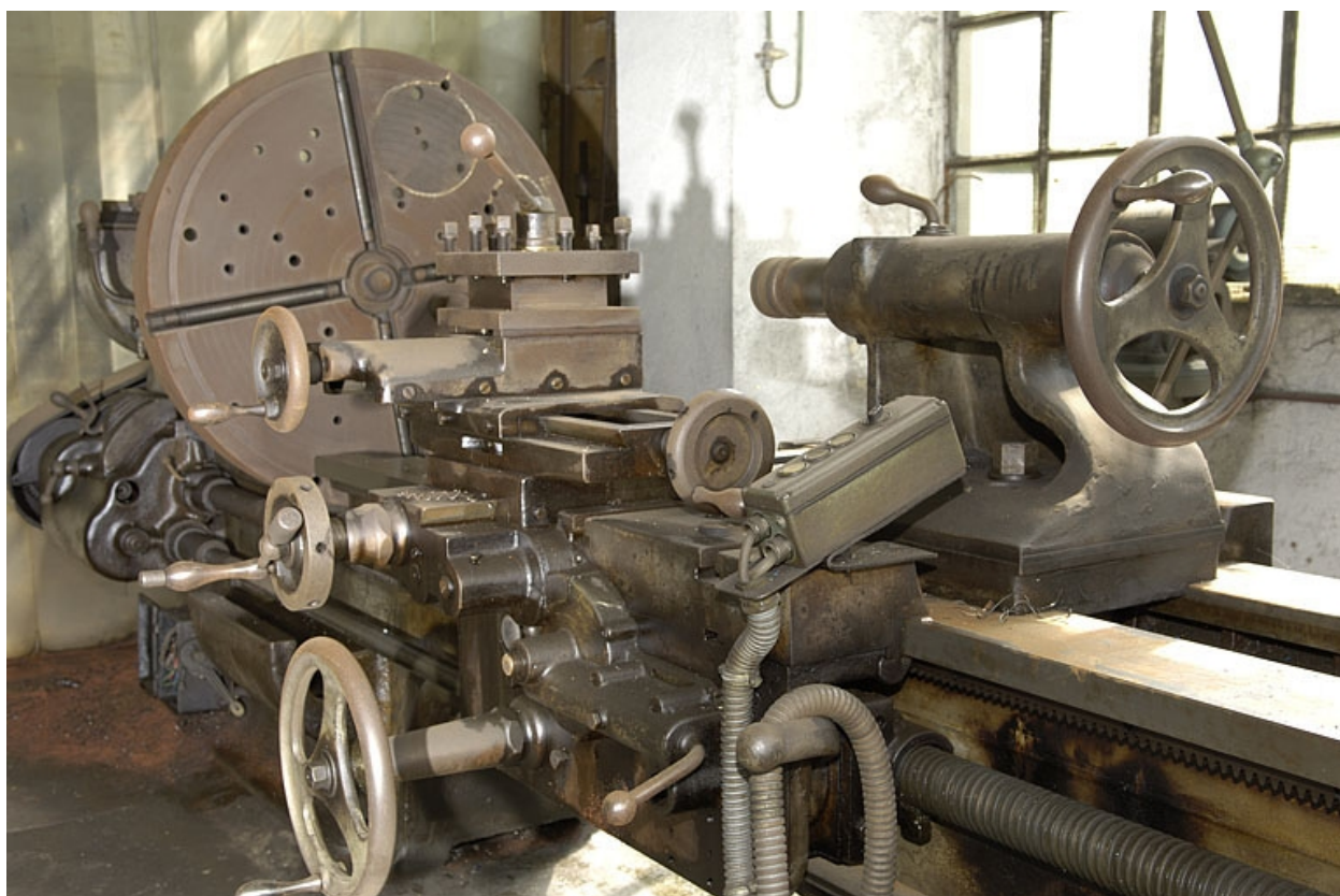
machine à tourner (tour à charioter et à fileter) : détail du chariot.
