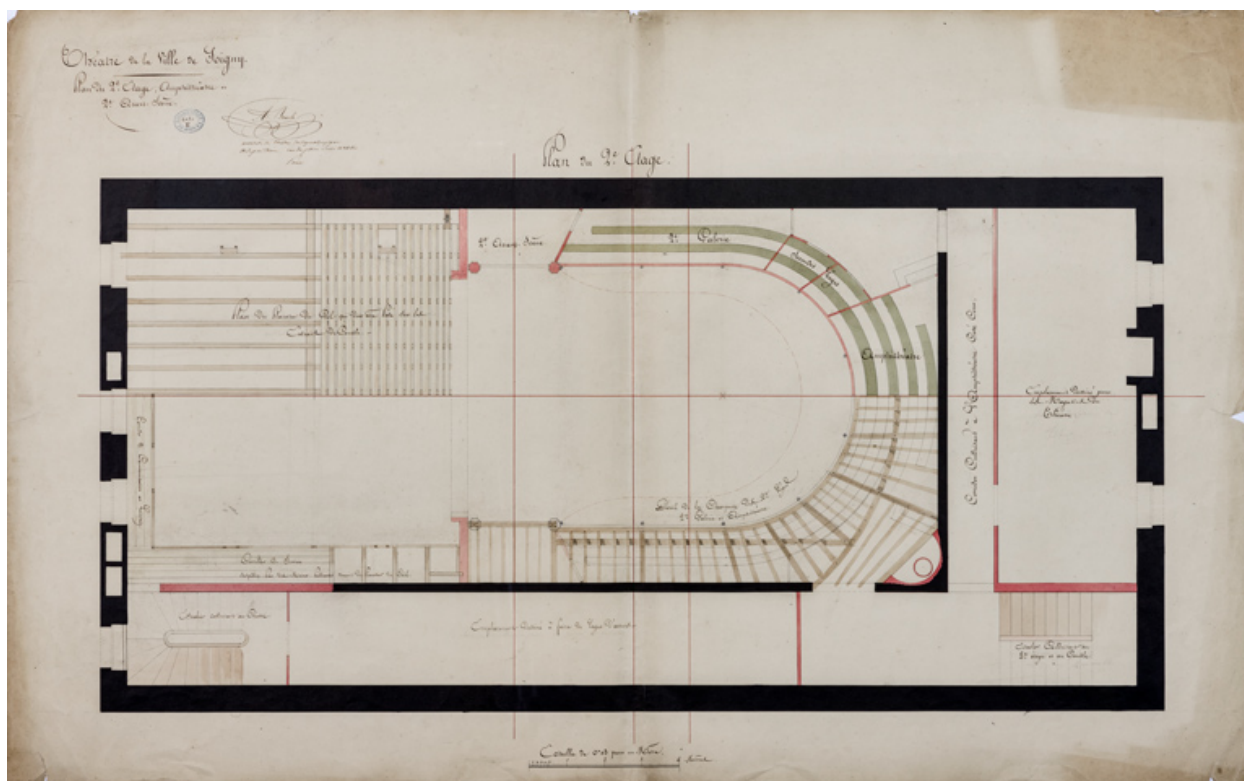
Construction de la salle de spectacle. Plan du 2e étage, amphithéâtre et 2e avant-scène. 1832.
