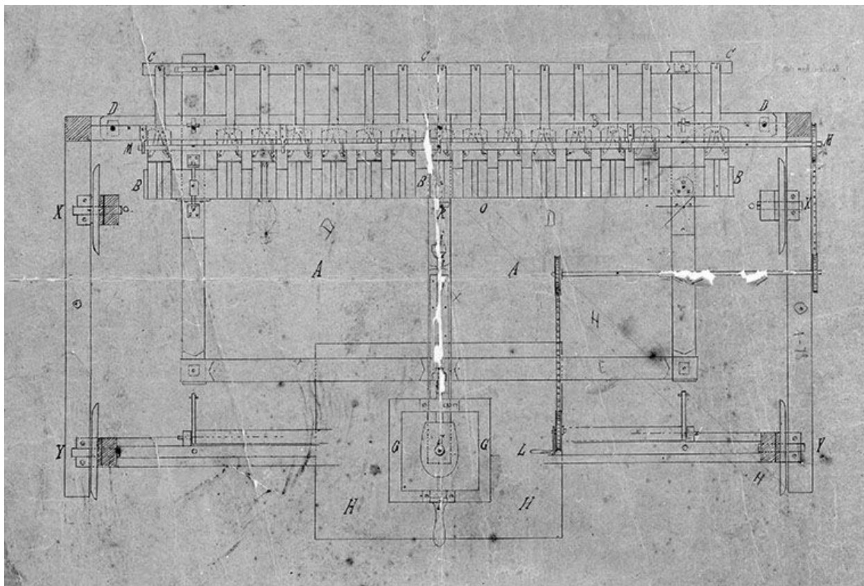
Plan de la machine.
