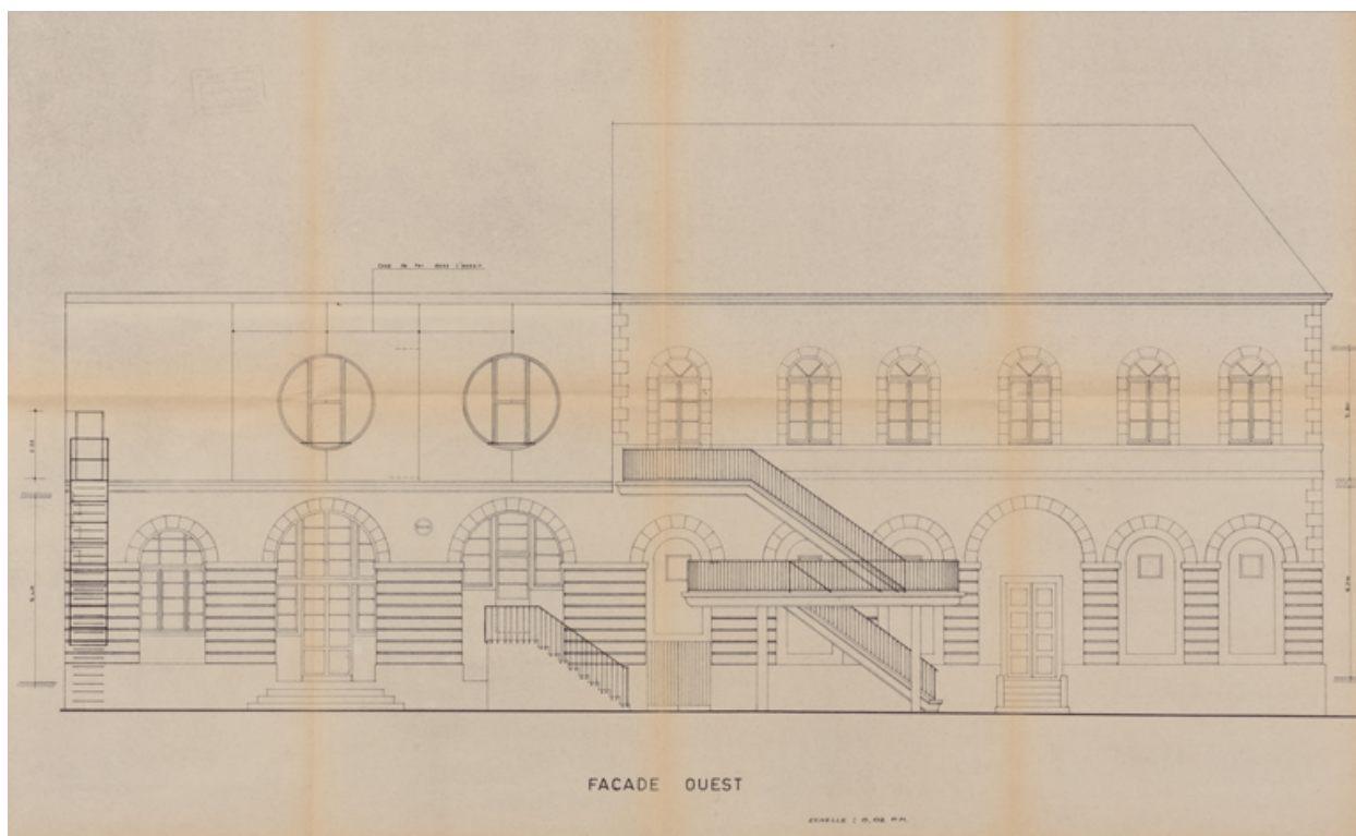
Ville de Prémery. Projet d'agrandissement de la salle des fêtes. 2. Façade ouest. Février 1970.
