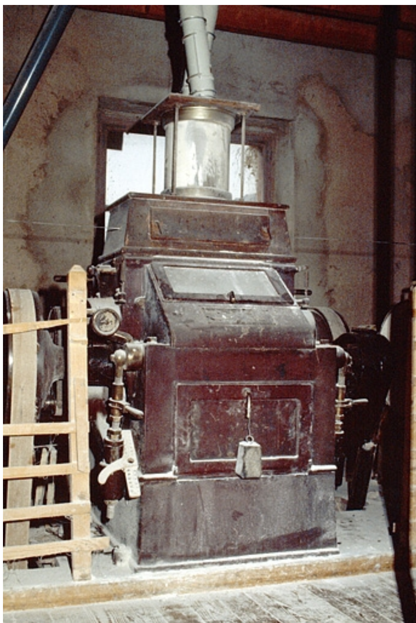
Minoterie (H), rez-de-chaussée : appareil à cylindres (convertisseur) Teisset-Rose-Brault.
