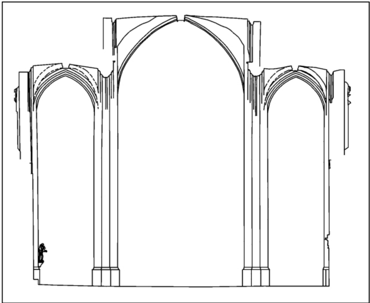
Restitution photogrammétrique d'une partie de la coupe transversale.
