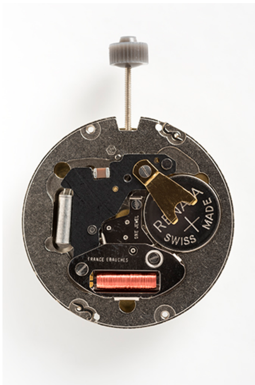
Mouvement France Ebauches FE 7221 : face côté fond.
