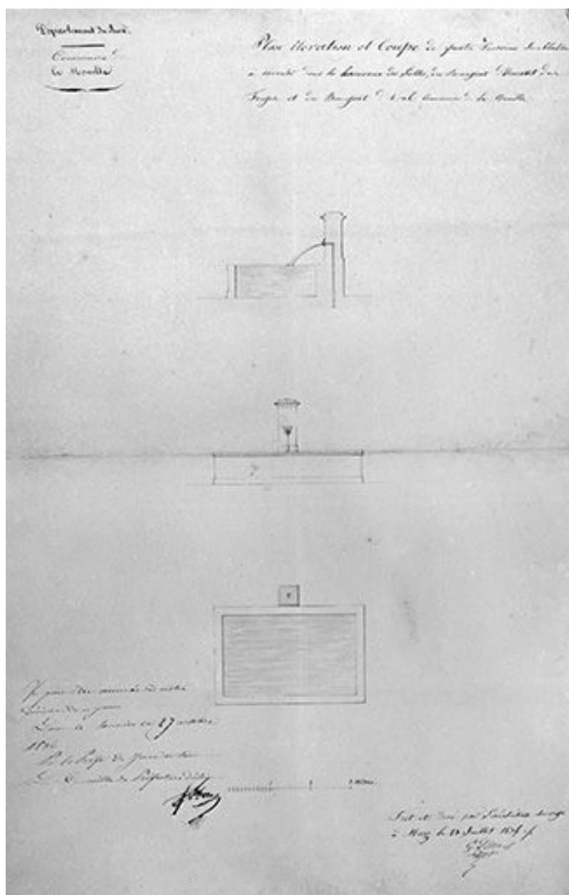
La Mouille : Plan, élévation et coupe de quatre fontaines semblables, 1836.
