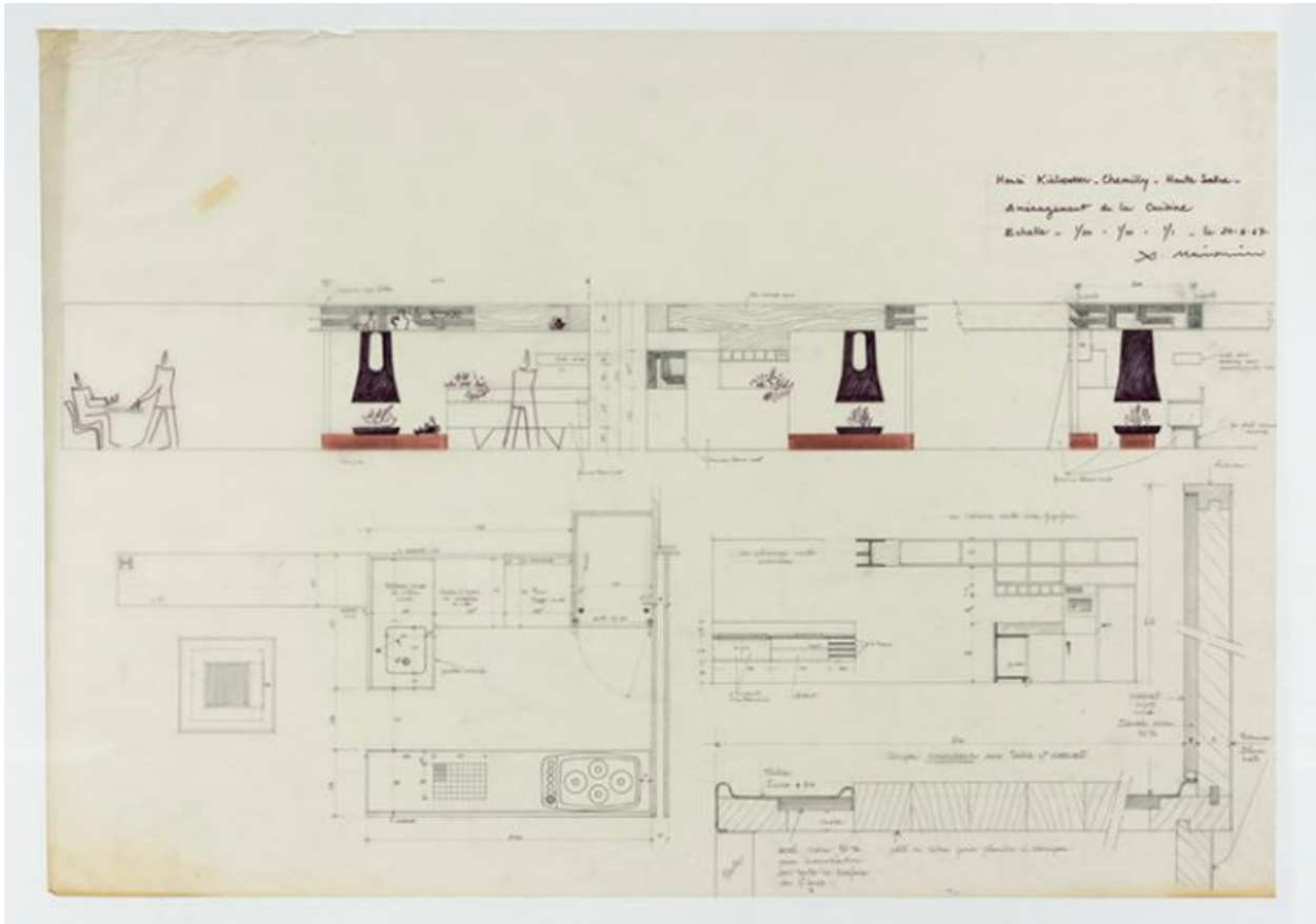
Plans et schémas d'aménagement de la cuisine.
