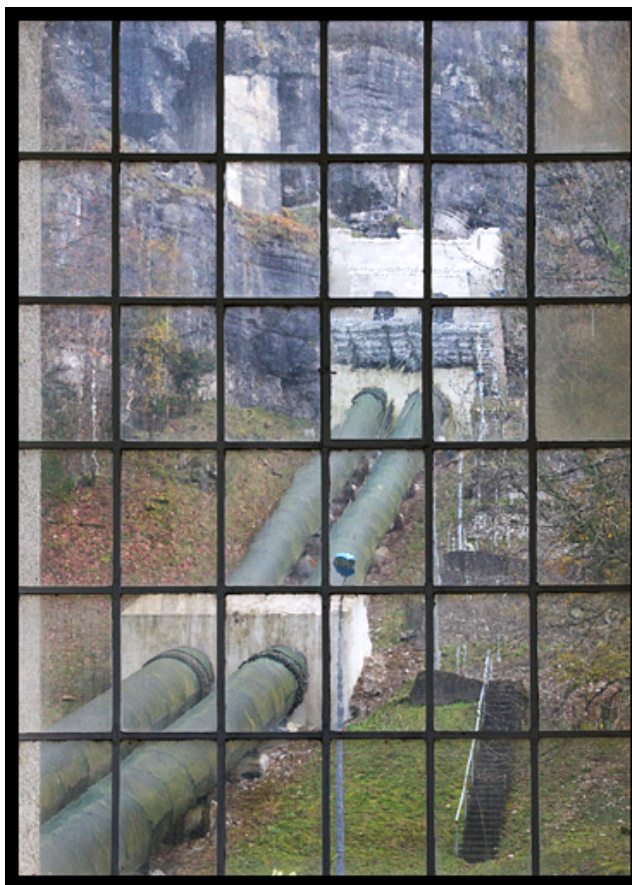
Centrale hydroélectrique du Refrain, Charquemont : conduite forcée, vue depuis l'intérieur de la salle des machines.
