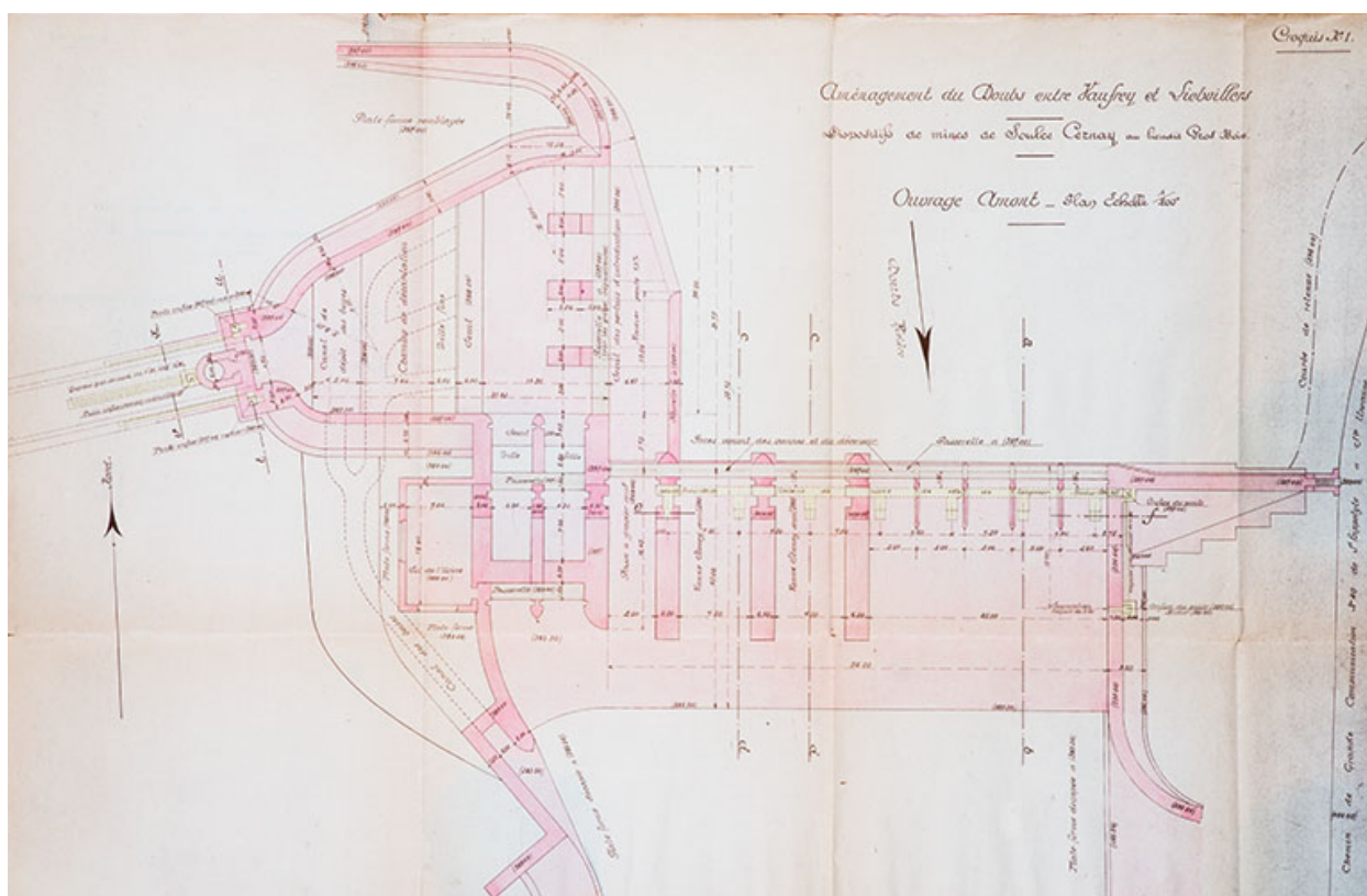
Aménagement du Doubs entre Vaufrey et Liebvillers. Dispositifs de mines de Soultz Cernay au lieu dit Gros Bois. Croquis n° 1. Ouvrage amont. Plan, 1924.
