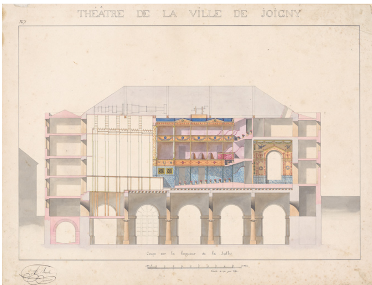
Coupe sur la longueur de la salle. N° 7. S.d. [1829-1830]. (MAP : G/82/89/2008-039062)
